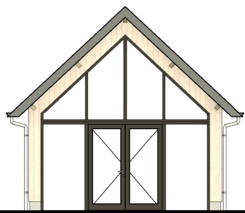
zuidgevel
